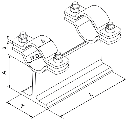
Industrierohrschellen DIN 3657 A Alle Maße in mm
